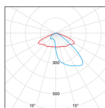
ÓPTICA II MEDIA
