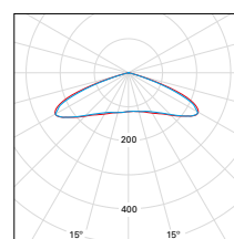
ÓPTICA V SIMÉTRICA
