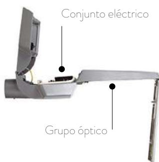
Equipo y grupo lumínico LED en un único cuerpo con dos cuerpos independientes
