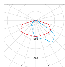
ÓPTICA III MEDIA*
